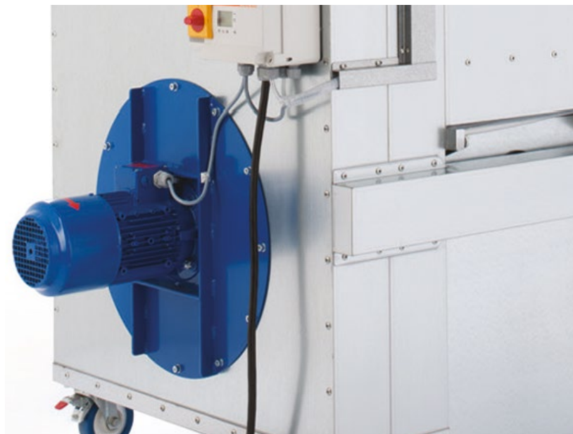
Abb. oben: Vacumobil VT 160 mit energieeffizientem 2,2 kW IE3-Motor
