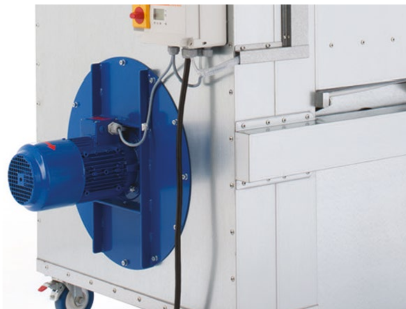
Abb. oben: Vacumobil VT 160 mit energieeffizientem 2,2 kW IE4-Motor
